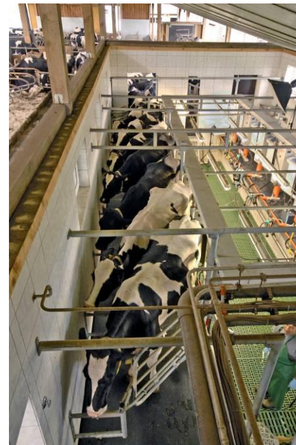
Blick ins „Schiebedach“ des Fischgrät-Melkstands.
